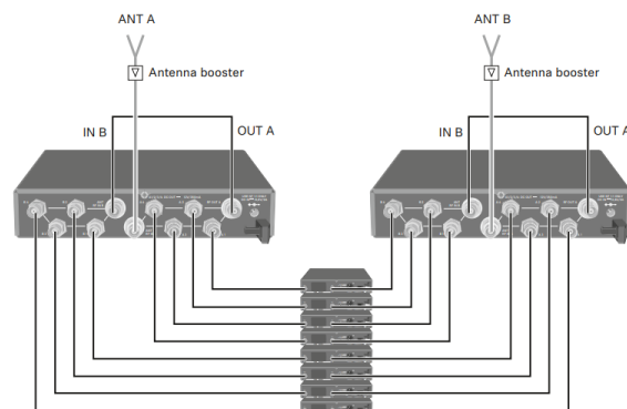
2台使用で8台のRF分配が可能
